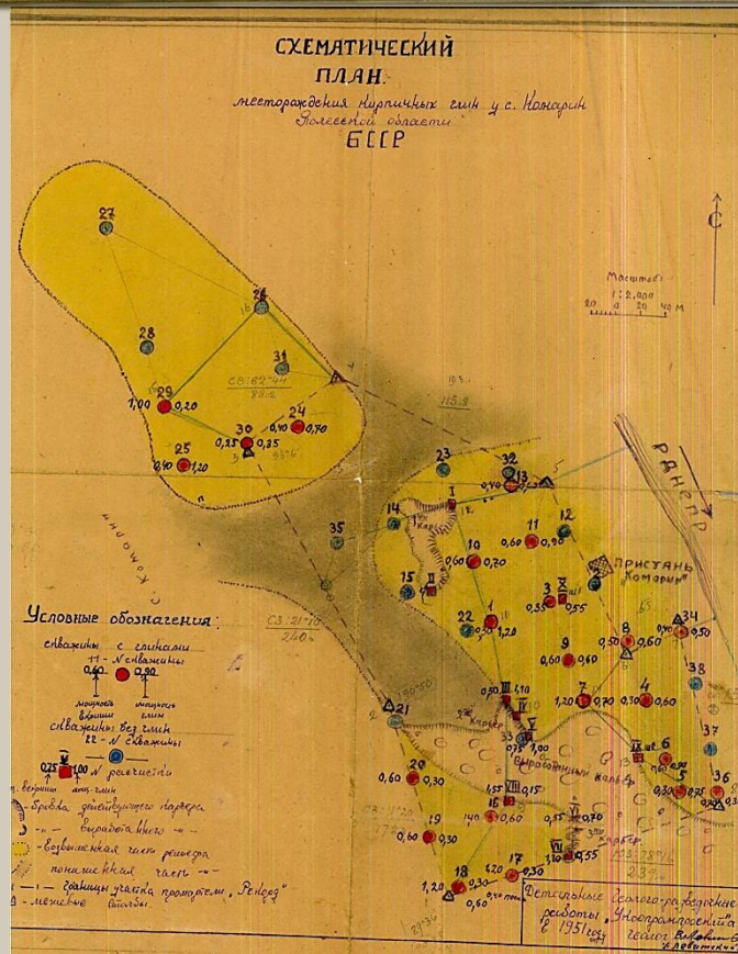
Схематический план месторождения кирпичных глин у д. Комарин. 1951 г. ЗГА в г. Речице. Ф. 118. Оп. 1. Д. 6. Л. 11
