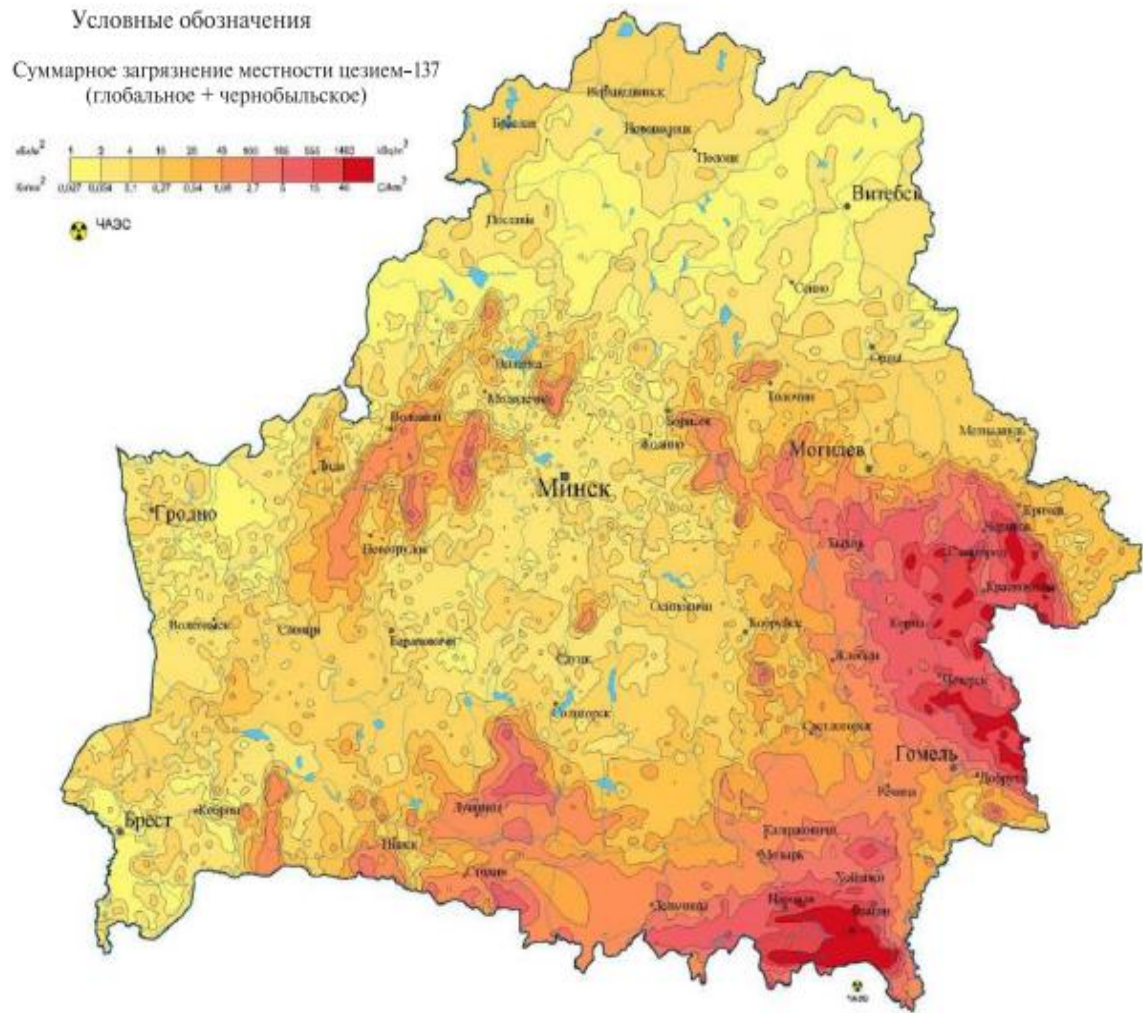
Рис. 1.2. Загрязнение территории Республики Беларусь цезием-137, по состоянию на 1986 г.
