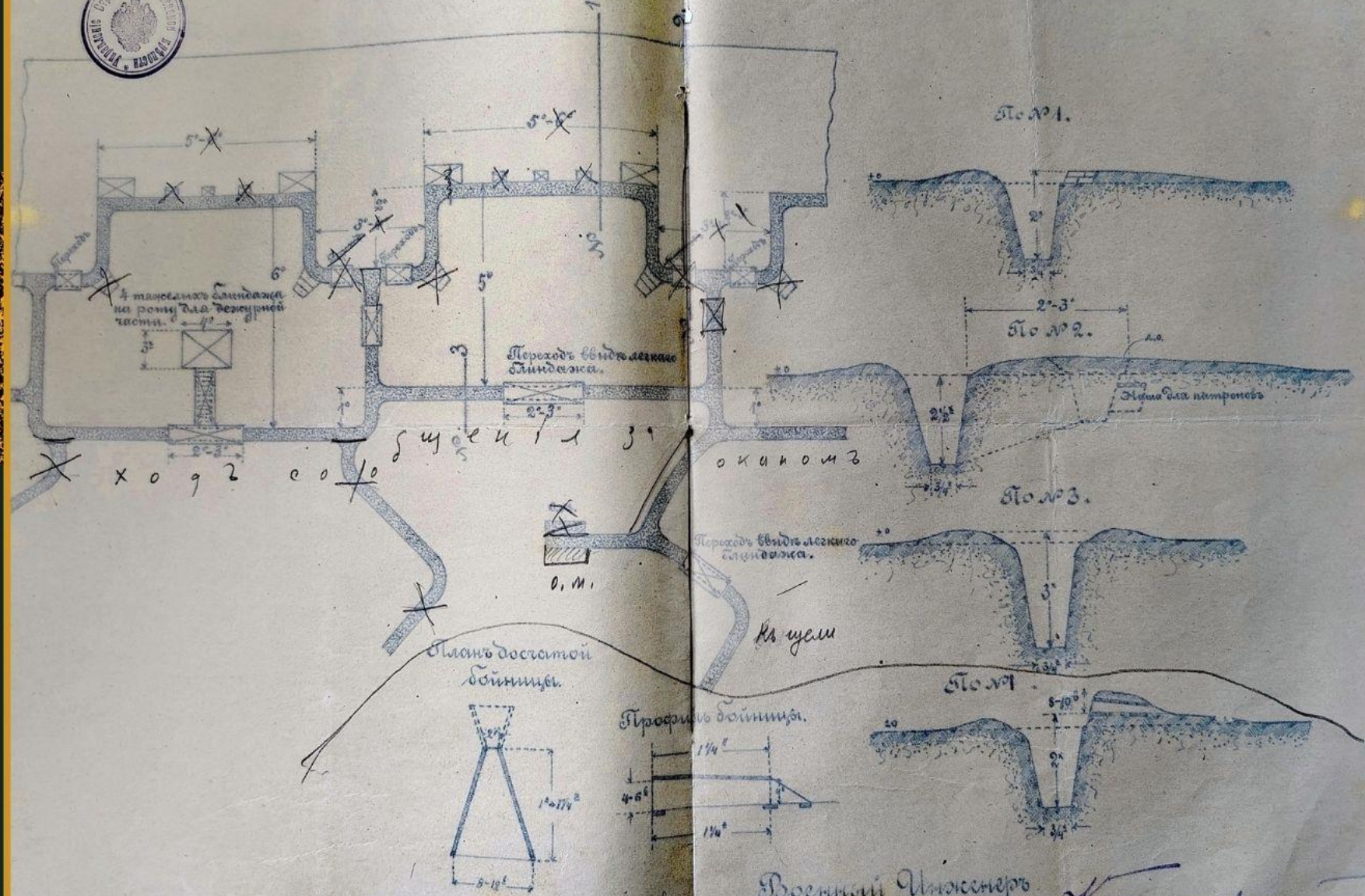
План стрѣлковаго окопа Гродненской крепости Гродненскаго уѣзда Гродненской губернии. Составлен военным инженером Колосовским, 8 октября 1915 г. Ф.731. Оп. 1. Д. 10. Лл. 17 об.-18.
