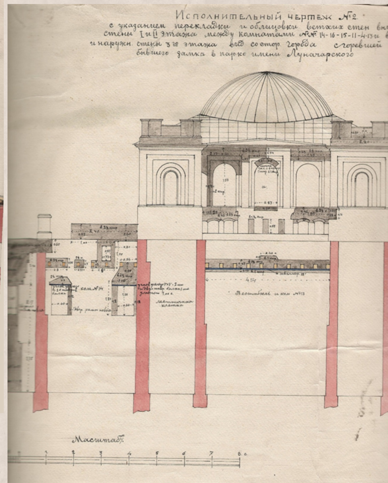
«Исполнительный чертеж № 1, 2, 3. Вид со стороны города сгоревшей части бывшего замка в парке имени Луначарского». 19 марта 1926 г.
