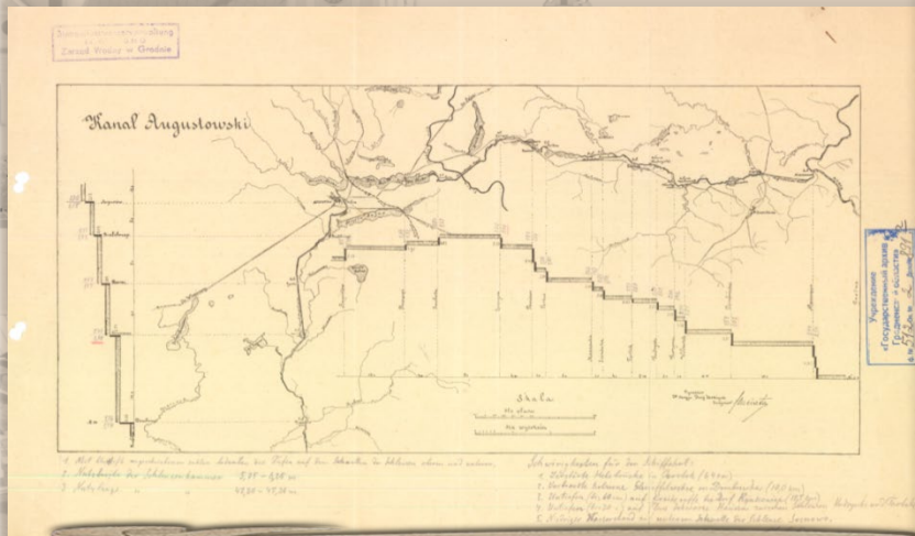
Чертёж Августовского канала. Не датирован. Ф. 512. Оп. 2. Д. 891 а.
