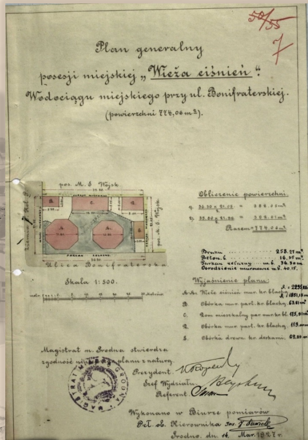
План водонапорных башен по ул. Бонифратерской (ныне Свердлова) в г. Гродно. 14.03.1927. Ф. 46. Оп. 1. Д. 190. Л. 7.
